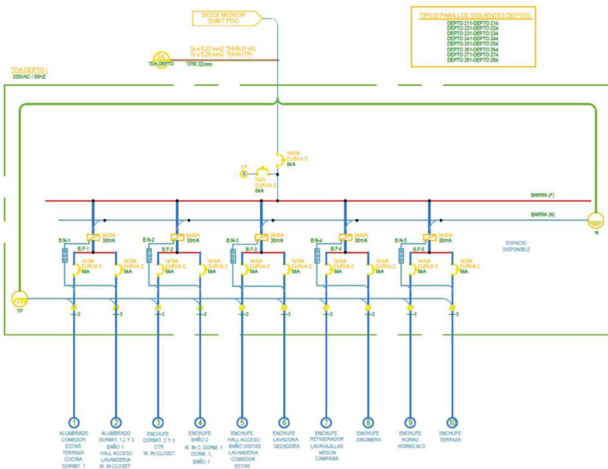
Imagen 2: Esquema unilineal depts. Tipo 1 y 4 (piso 1 al 8)
