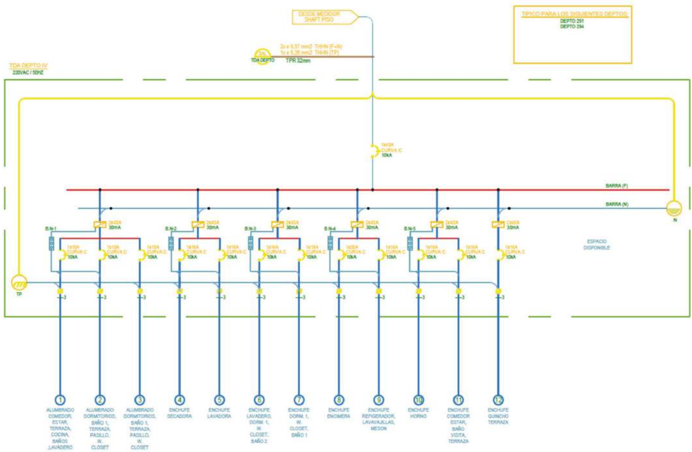
Imagen 4: Esquema unilíneal depts. Tipo 1 y 4 (piso 9)
