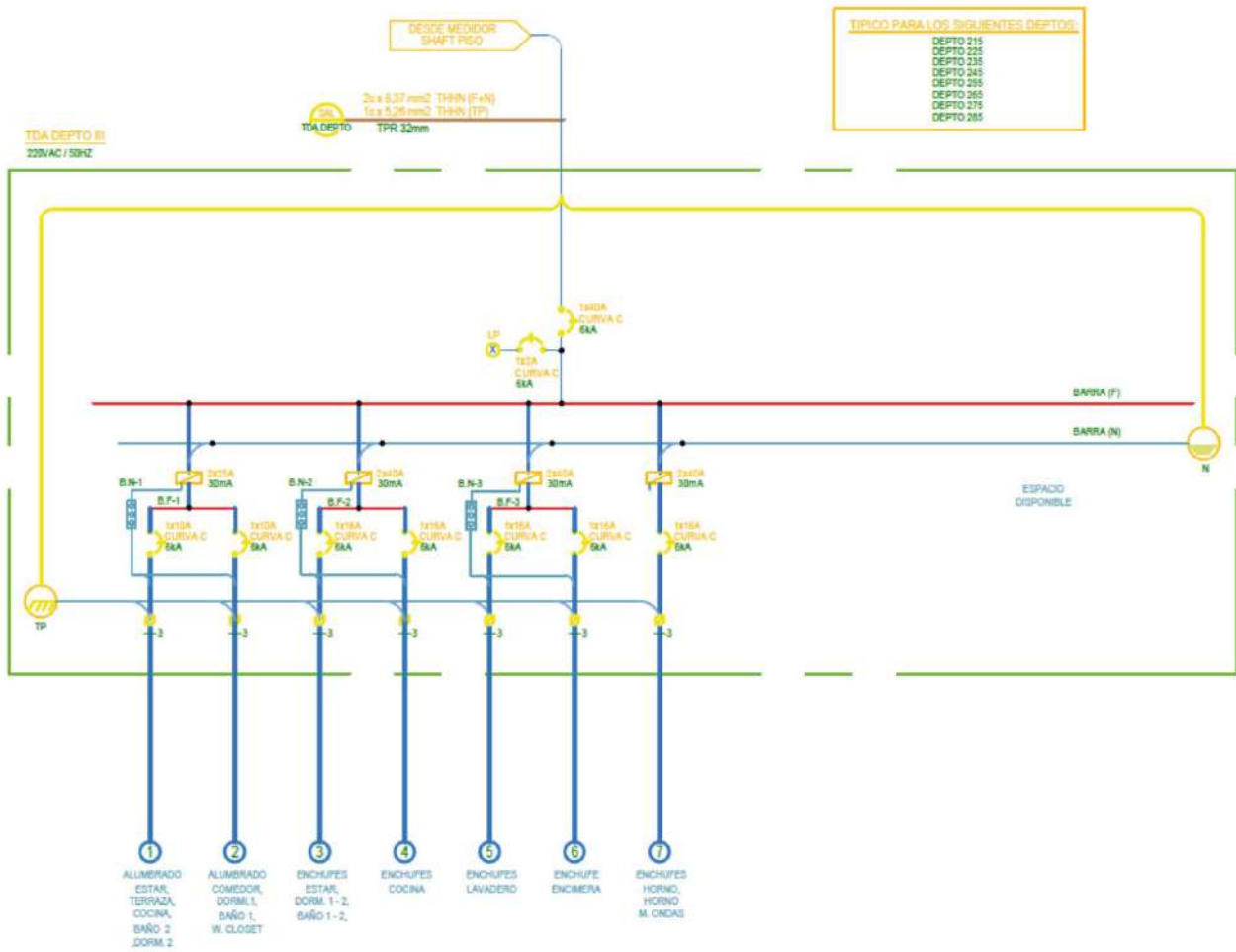
Imagen 3: Esquema unilineal deptos. Tipo 5
