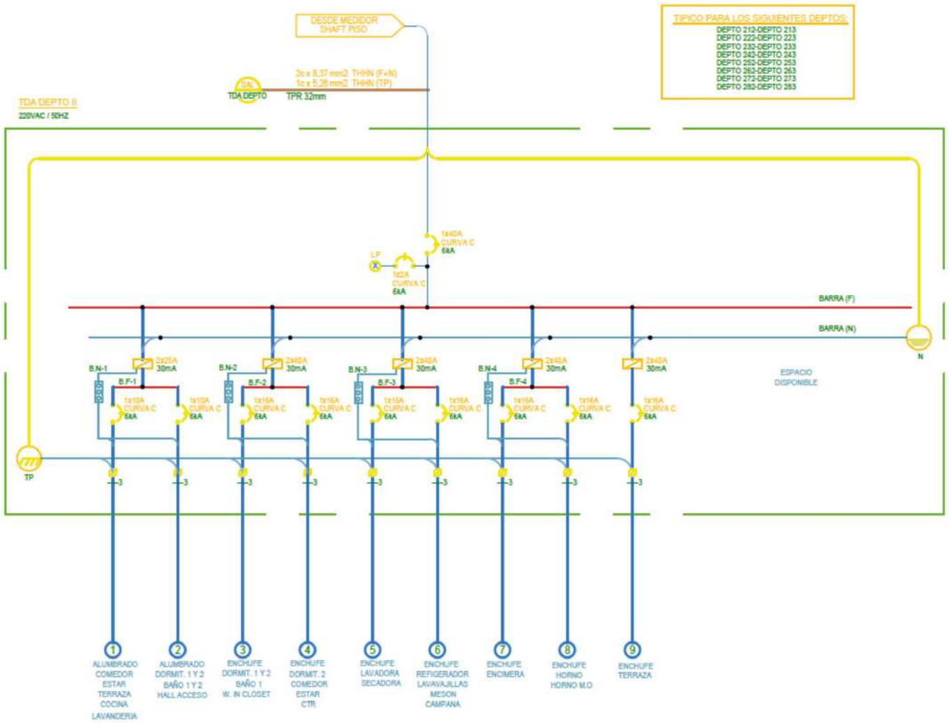
Imagen 1: Esquema unilineal Deptos. Tipo 2 y 3
